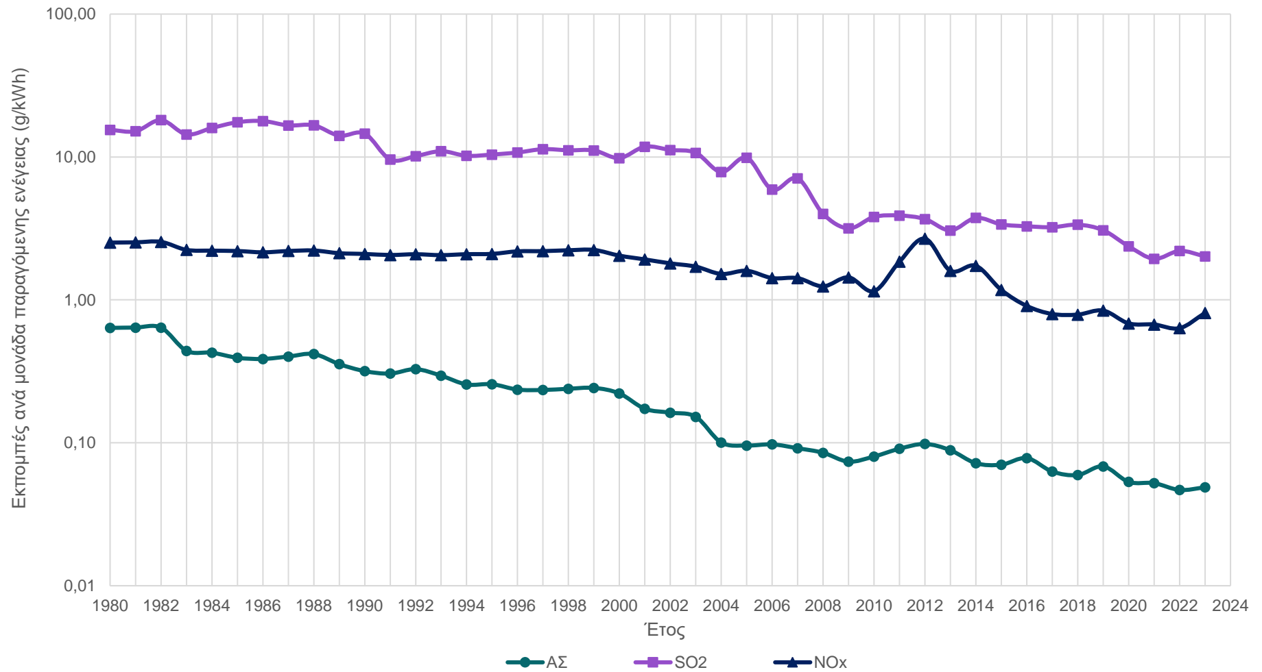
Γράφημα - Ετήσια διακύμανση περιβαλλοντικών δεικτών εκπομπών ΑΣ, SO 2 , NO x σε γραμμάρια ανά κιλοβατώρα από συμβατικές μονάδες ηλεκτροπαραγωγής μεγάλης κλίμακας (λογαριθμική κλίμακα)
